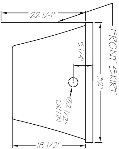
END ELEVATION
